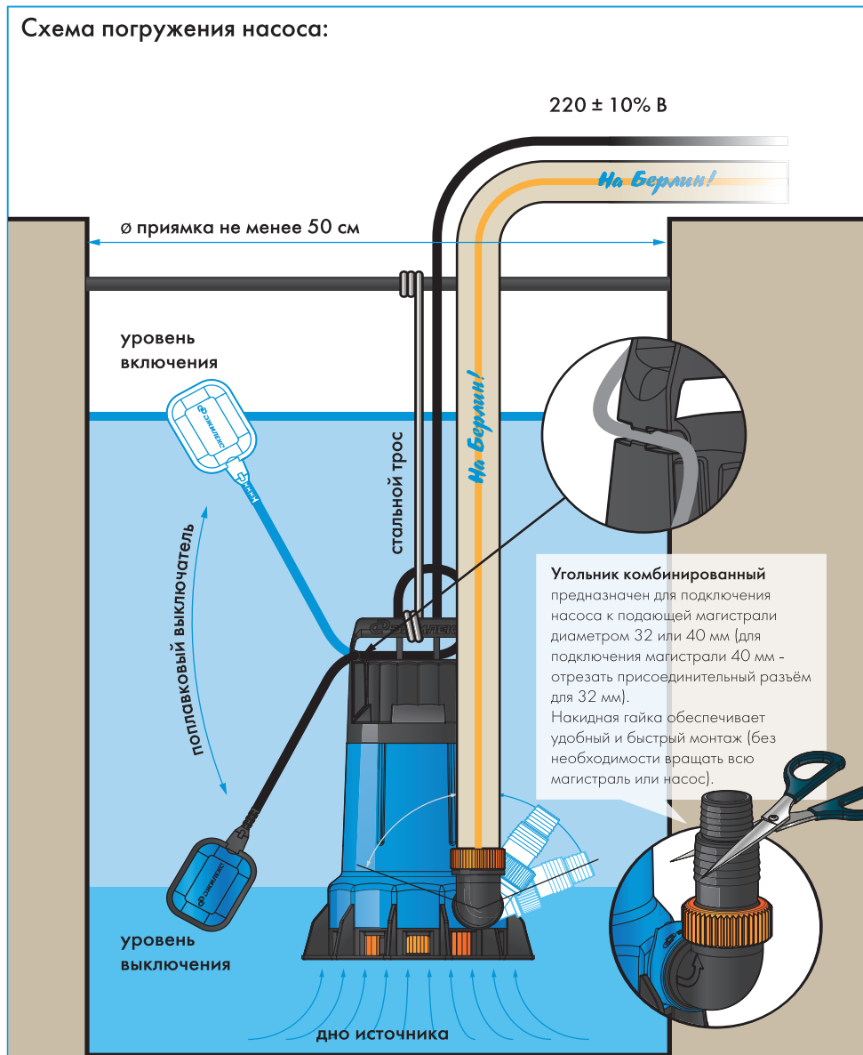
Рисунок 3 (на примере изображен насос погружной «ДРЕНАЖНИК» 350/17).
